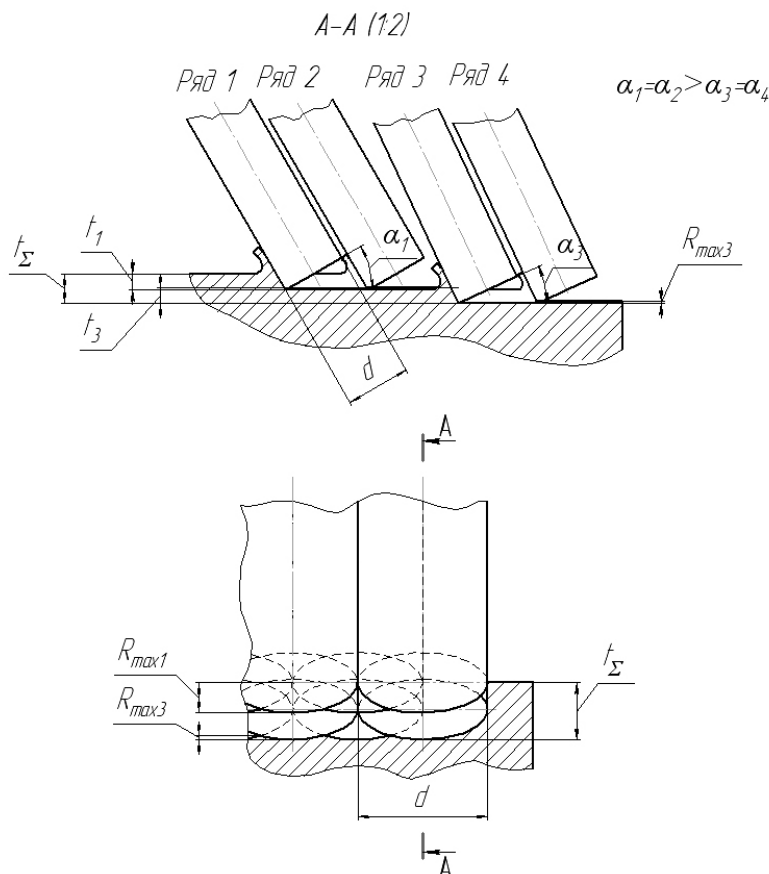
Рисунок 1 — Расчетная схема процесса иглофрезерования плоской поверхности
