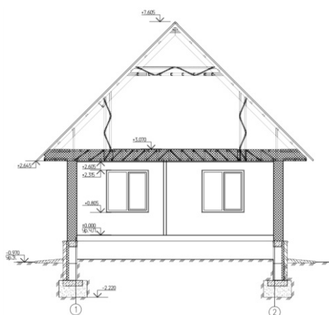
Рисунок 3. Разрез
