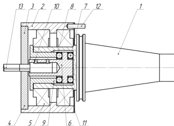
Рисунок 1 — Оснастка для обработки отверстий квадратного сечения
