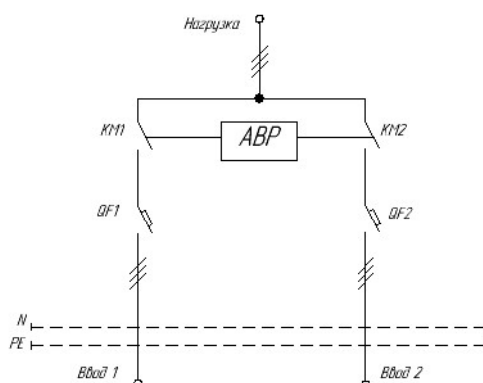
Рисунок 1 - Однолинейная схема АВР
