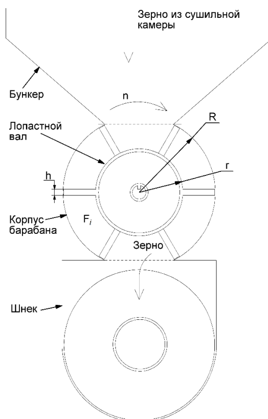
Схема расположения питателя-распределителя в ЭАПЗ
