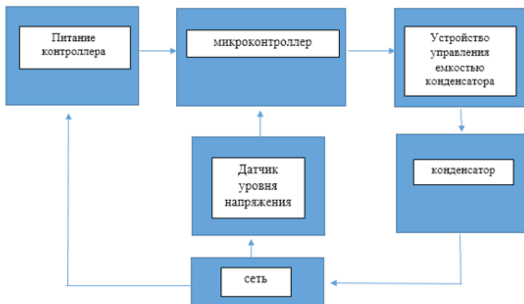
Блок-схема устройства для повышения напряжения в конце линии
