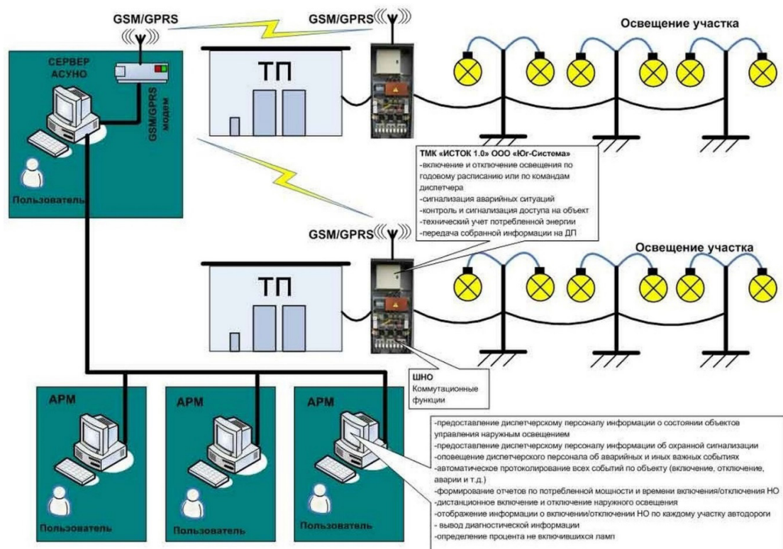
Структура автоматизированной системы управления уличным освещением
