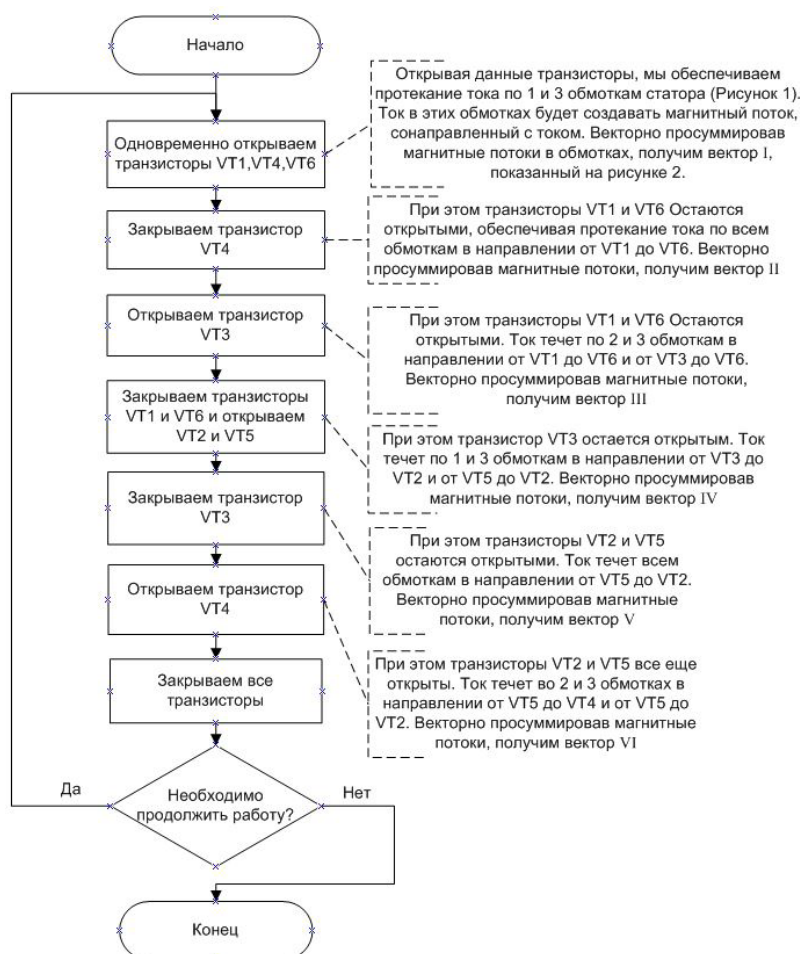
Алгоритм работы схемы ЧП с ВАУ
