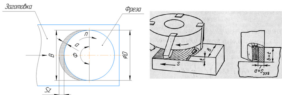
Рисунок 1 — Ширина срезаемого слоя (а) при торцевом фрезеровании
