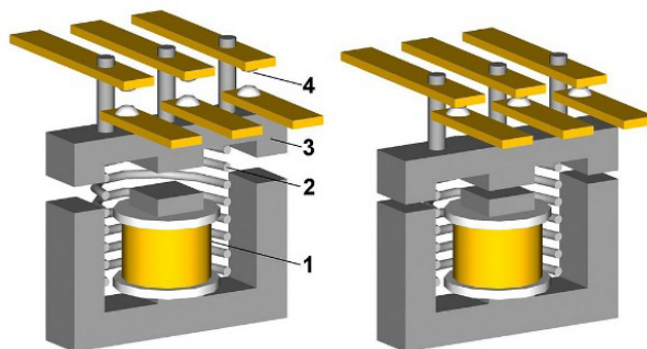
1 — катушка; 2 — пружина; 3 — подвижная часть; 4 — замыкающие контакты Рисунок 1 — Принципиальная схема конструкции трехфазного контактора
