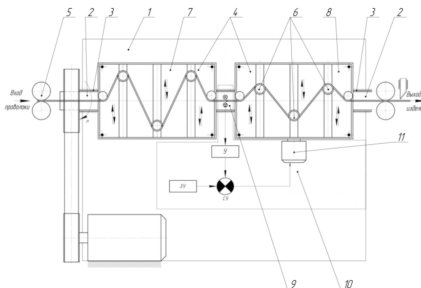
Рисунок 1 — Устройство для правки и гибки проволоки
