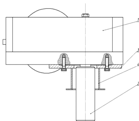
Рисунок 1 — Крепление редуктора до модернизации: 1 — мотор-редуктор; 2 — вал-хвостовик; 3 — фланец; 4 — обсадная труба
