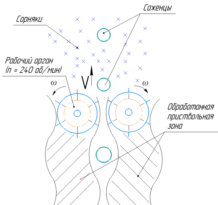
Рисунок — Схема обработки приствольной зоны одного ряда
