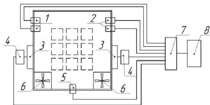
1, 2 - датчики влажности и температуры, 3 - магнетроны, 4 - программируемые реле, 5 - датчики давления, 6 - вентиляторы, 7 - модули ввода/вывода, 8 - контроллер
