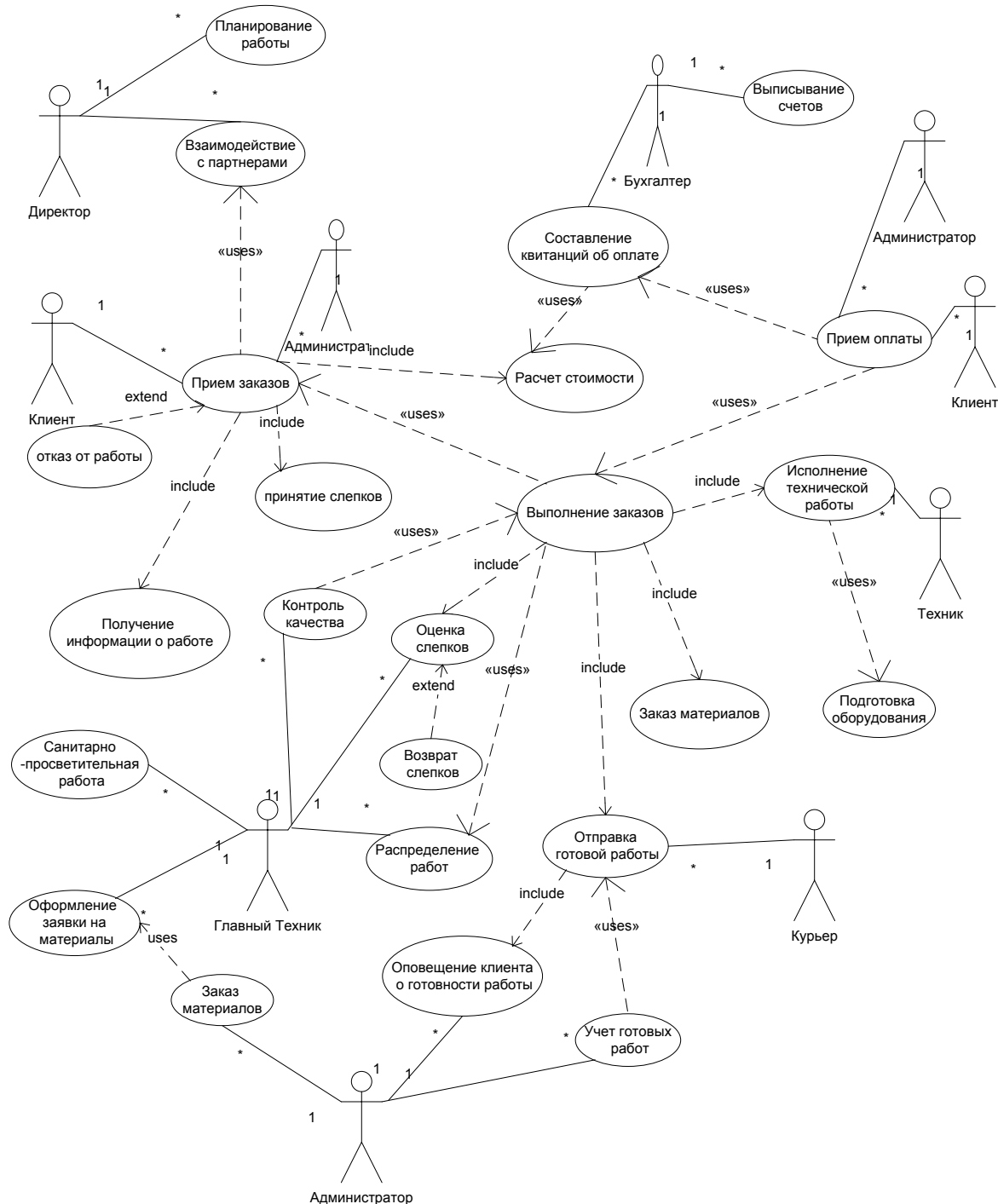
Рисунок 1 — Модель бизнес-прецедентов предметной области
