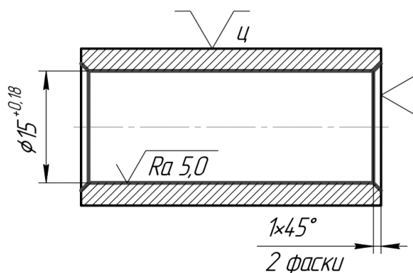
Рисунок 1 — Операционный эскиз обработки отверстия втулки
