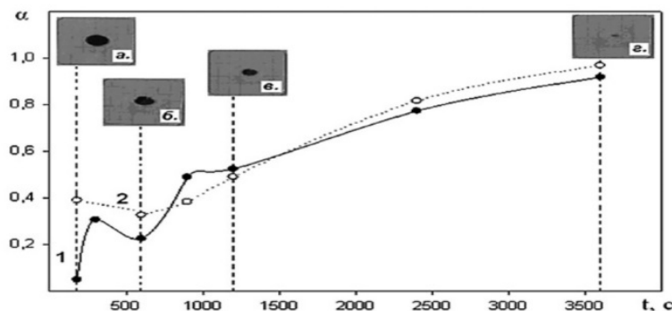
Рисунок 1. Кинетика окисления тонких пленок: 1 — пленка с удельной электропроводностью 3.3 \times 10^5 МСм/м, 2 — пленка с удельной электропроводностью 3.7 \times 10^5 МСм/м
