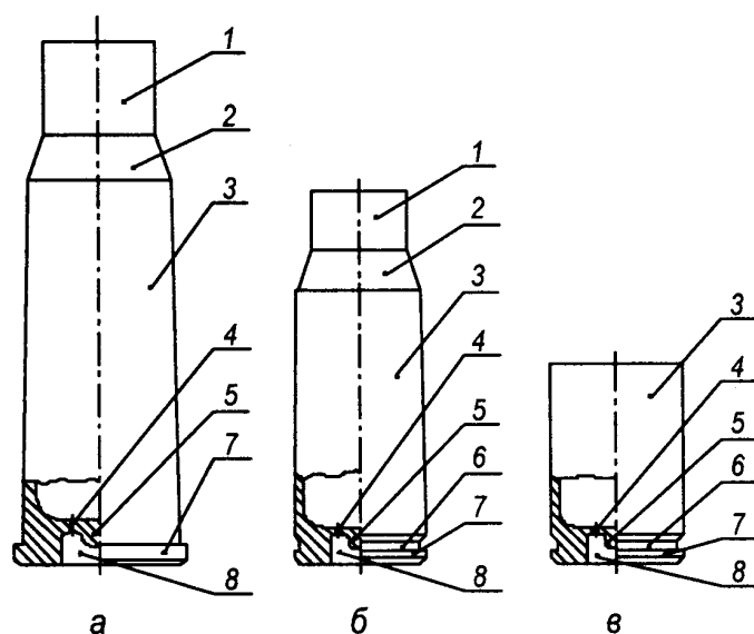
Рис. 1 Образцы гильз: а – винтовочная с выступающим фланцем; б – автоматная с проточкой; в – пистолетная цилиндрическая; 1 – дульце; 2 – скат; 3 – корпус; 4 – запальное отверстие; 5 – наковальня; 6 – проточка; 7 – фланец; 8 – капсюльное гнездо
