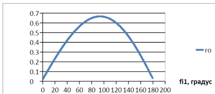
Рисунок 2. График зависимости ширины срезаемого слоя от углового положения зуба
