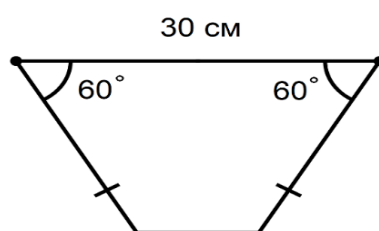
Рис. 1. Форма модернизированного вентиляционного канала
