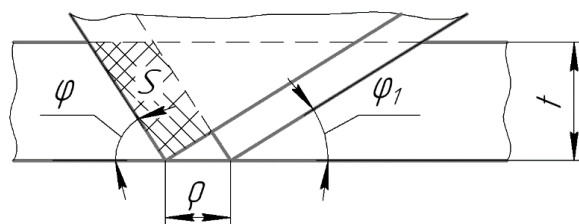
Рисунок 2. Положения двух последовательных зубьев
