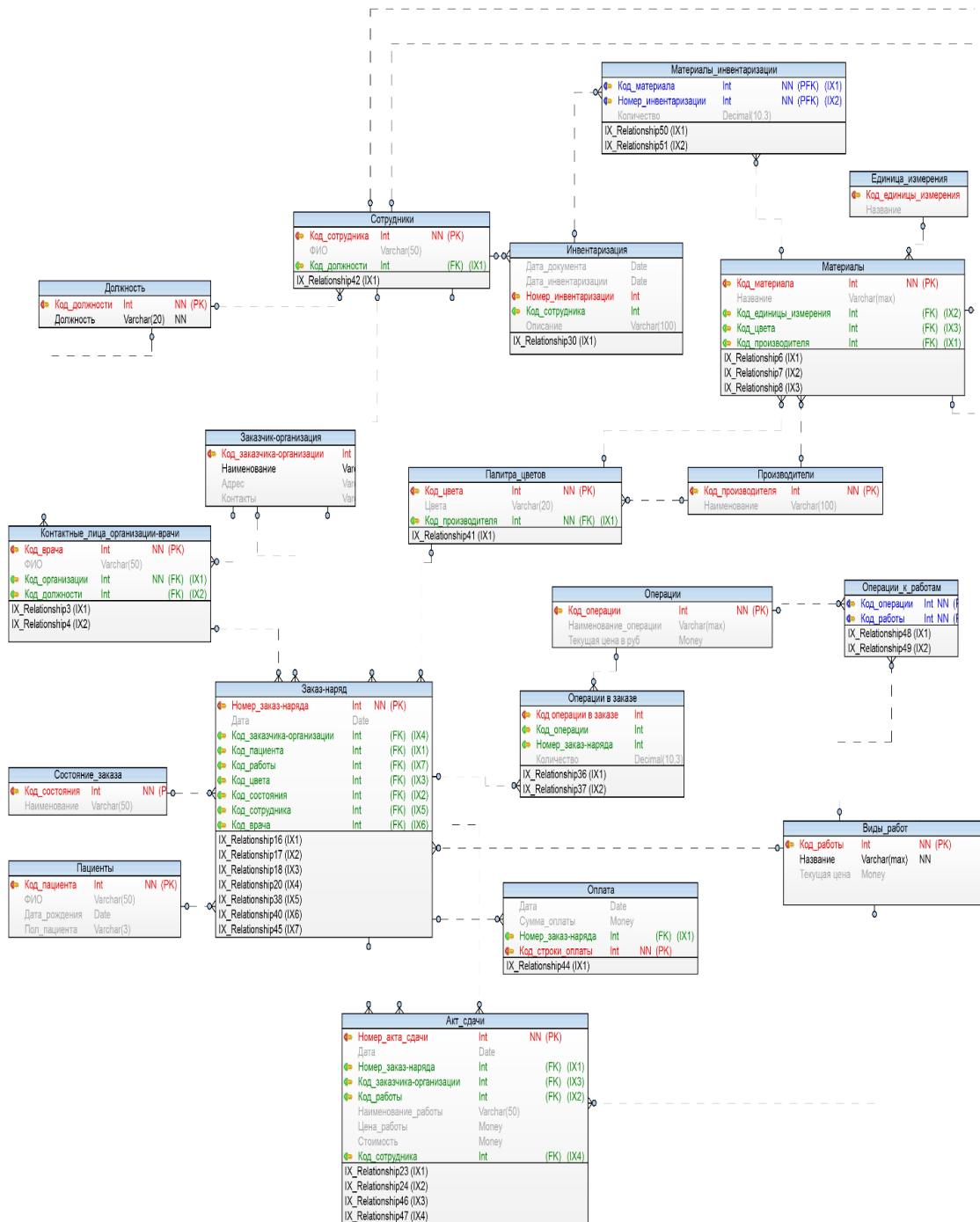
Рисунок 2. – Фрагмент логической схемы базы данных
