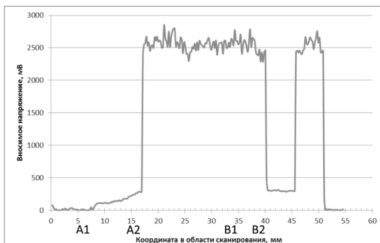
Рисунок 1 — Зависимость вносимого напряжения от координаты сканирования. A1-A2 — границы первого дефекта (область 1), B1-B2 — границы второго дефекта (область 3)
