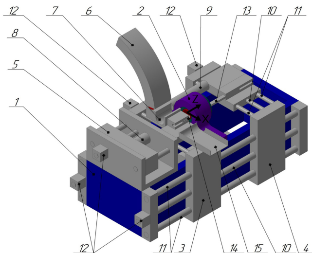
Рисунок 2 — 3D модель станка
