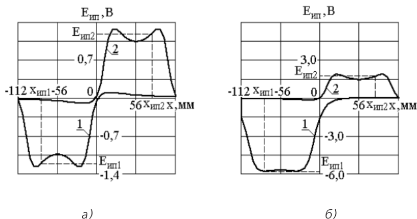
Рисунок 2 — ЭДС индукционных преобразователей при номинальной нагрузке и при витковом замыкании
