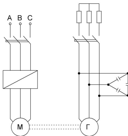
Рисунок 1 — Электрическая схема стенда для тестирования
