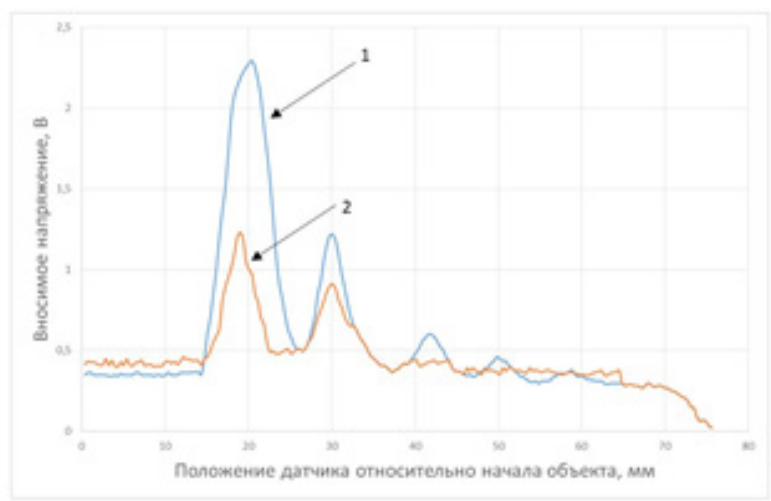
Рис. 1. Результаты сканирования пластины с использованием двух ВТП
