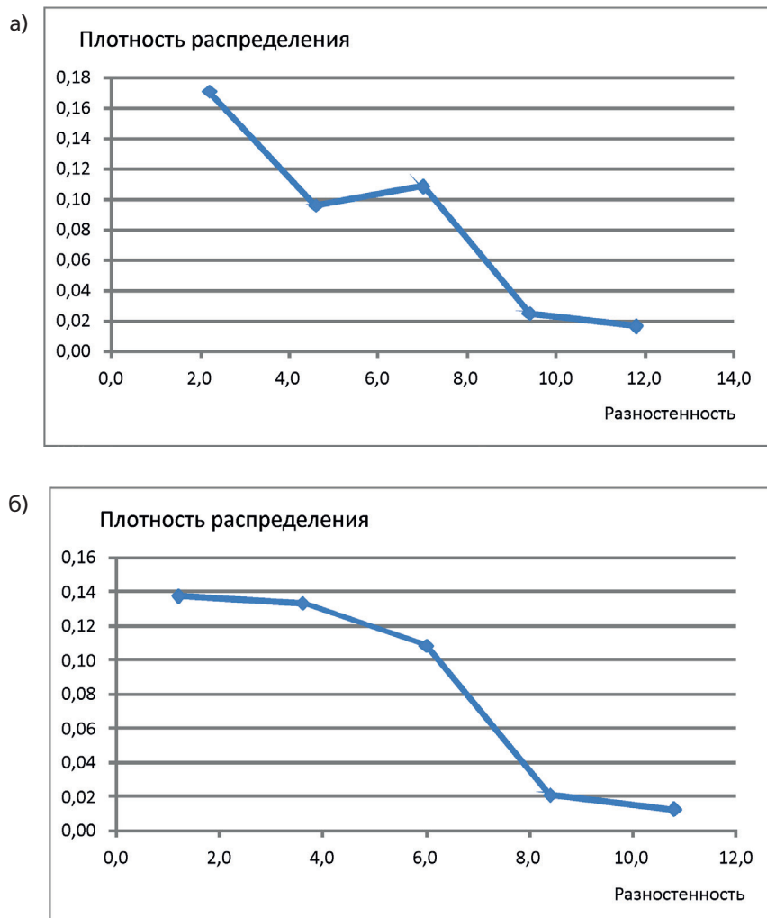
Рисунок 3 — Полигон распределения величины разностенности после второй вытяжки (а — дно гильзы, б — обрез гильзы)
