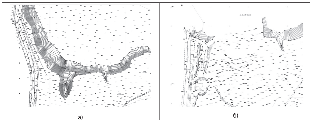
Рисунок 1 — Фрагменты топографических планов полигона ТБО: а) по результатам съемки 2011 г.; б) по результатам съемки 2019 г.
