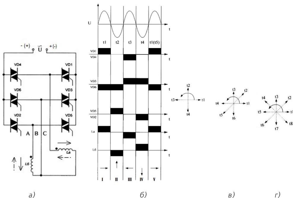
Рисунок 1 – Симисторный редуктор, ведомый сетью однофазного переменного напряжения, для двухфазного асинхронного двигателя, и его работа:
