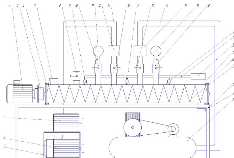
Рисунок — Экспериментальная установка для увлажнения зерна.
