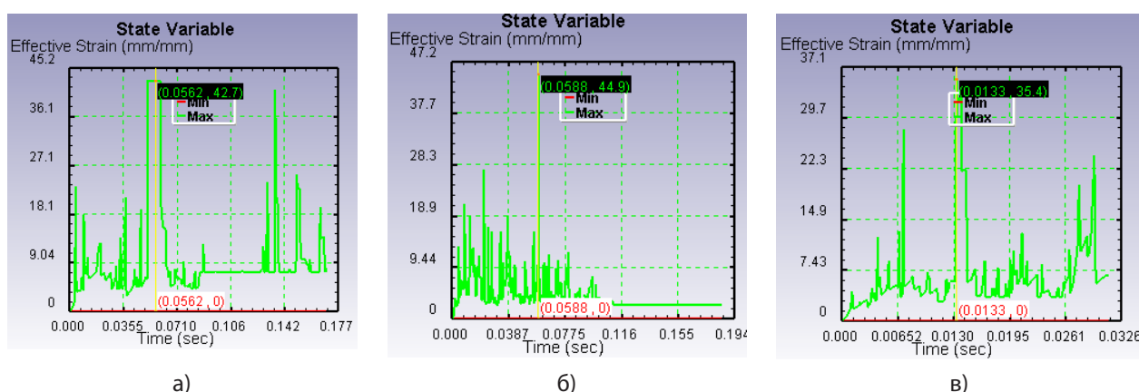
Рис. 2 — Максимальная деформация, возникающий в заготовке при точении: а — при v=50 ; б — v=100 ; в — v=150
