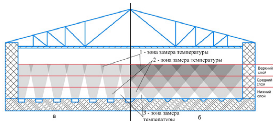
Рис. 2. Схема прохождения воздушных потоков через зерновой слой при использовании: а-прямоугольных каналах; б-трапециевидных каналах
