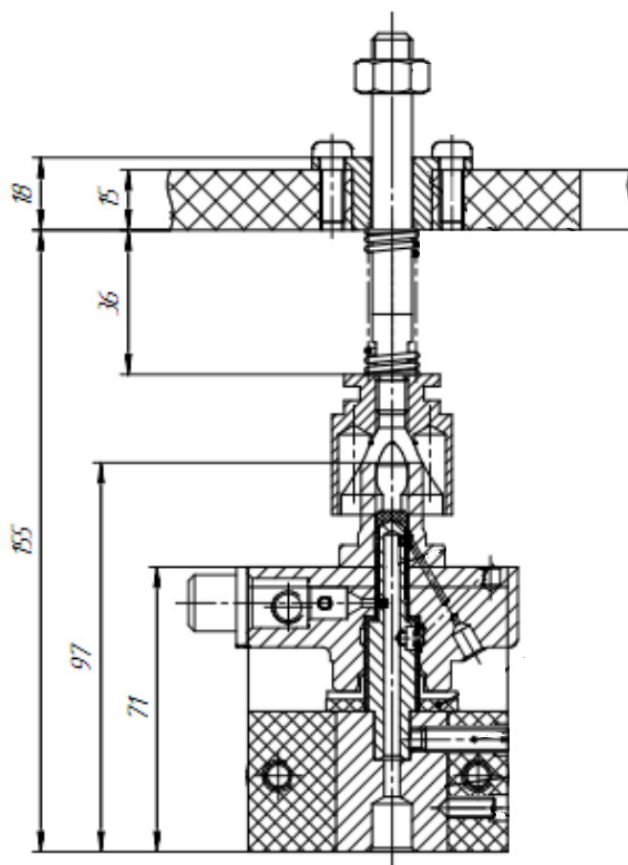
Рисунок 1 — Приспособление для электрохимической обработки втулки плунжера
