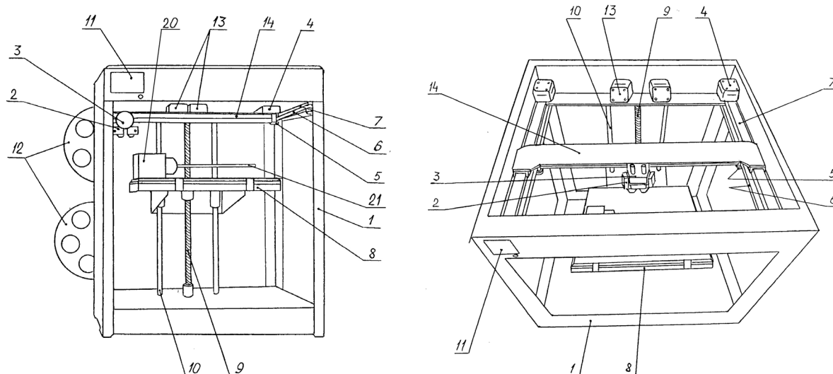
Рисунок 1—3D принтер с расширенными технологическими возможностями
