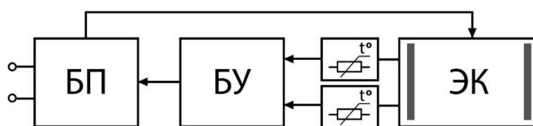
Блок-схема установки ЭК- обеззараживания
