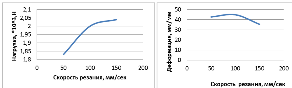
Рис.3 — Зависимость нагрузки от скорости резания Рис.4 — Зависимость деформации от скорости резания
