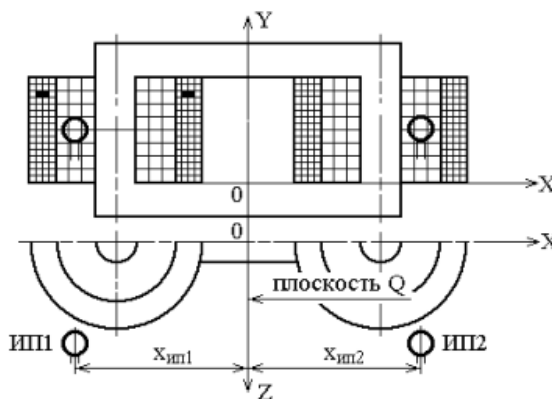
Рисунок 1 — Взаимное расположение элементов обмоток высокого и низкого напряжения трансформатора и измерительных преобразователей
