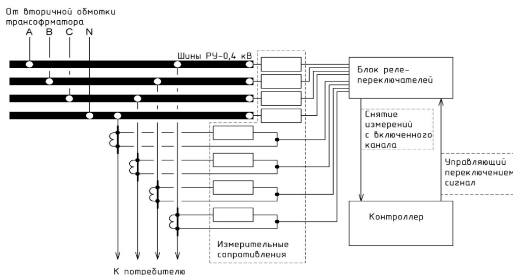
Рисунок 10 – Принципиальная схема процесса поочередного измерения параметров электроэнергии распределительной сети 0,4 кВ
