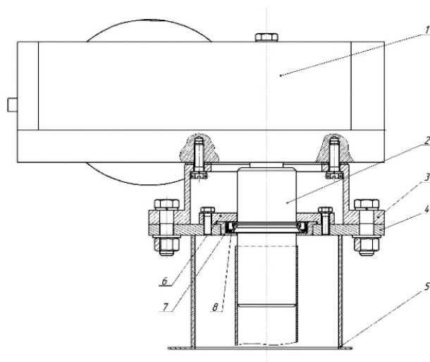
Рисунок 2 — Новое крепление редуктора: 1 — мотор-редуктор; 2 — вал-хвостовик; 3 — седло; 4 — фланец; 5 — обсадная труба; 6 — фланец манжеты; 7 — манжета; 8 — обойма
