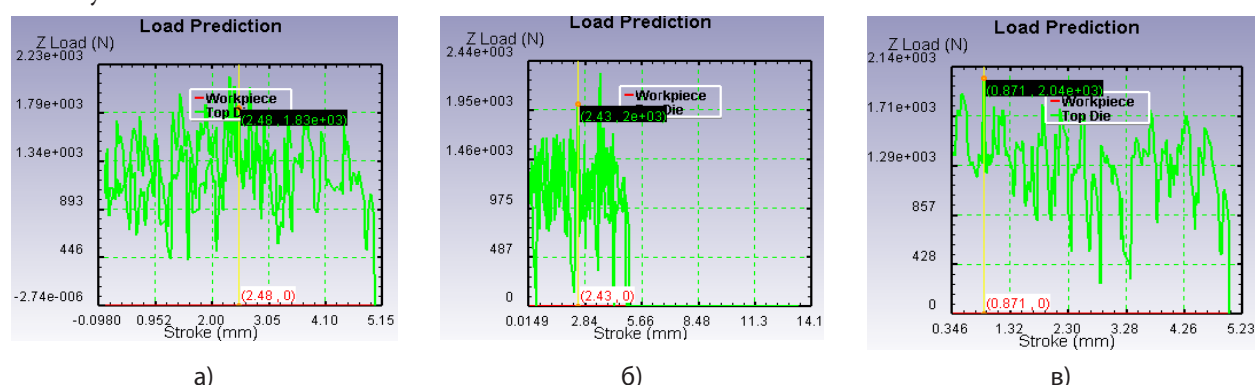
Рис. 1 — Максимальная нагрузка, возникающая в заготовке при точении: а — при v=50 ; б — v=100 ; в — v=150
