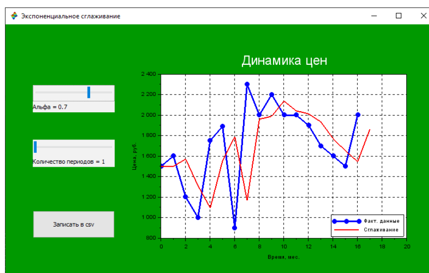
Рисунок 3 – Визуализация влияния параметра экспоненциального сглаживания Альфа на результаты аппроксимации и прогноза
